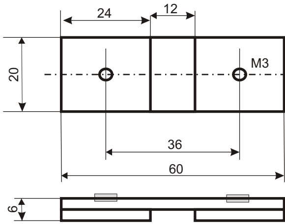
My Way Träger zu Regler vorn Ceiba Leichtbausperrholz 3 mm 16.12.17 PG
